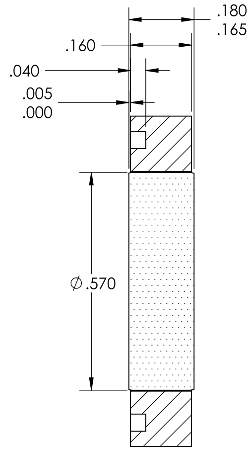
SECTION A-A
